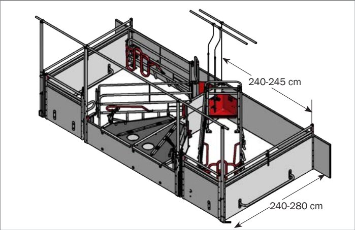
1. BOX PARTO CON PIANTONI ALTI Consigliato per box 240-245 cm C/C.
