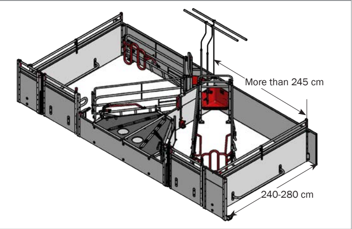
2. BOX PARTO CON PARTE ANTERIORE E MONTANTE BASSO Consigliato per box 245 cm c/c
